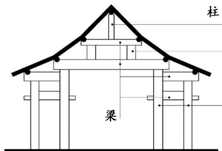
中国古建筑大木构架剖面示意图
